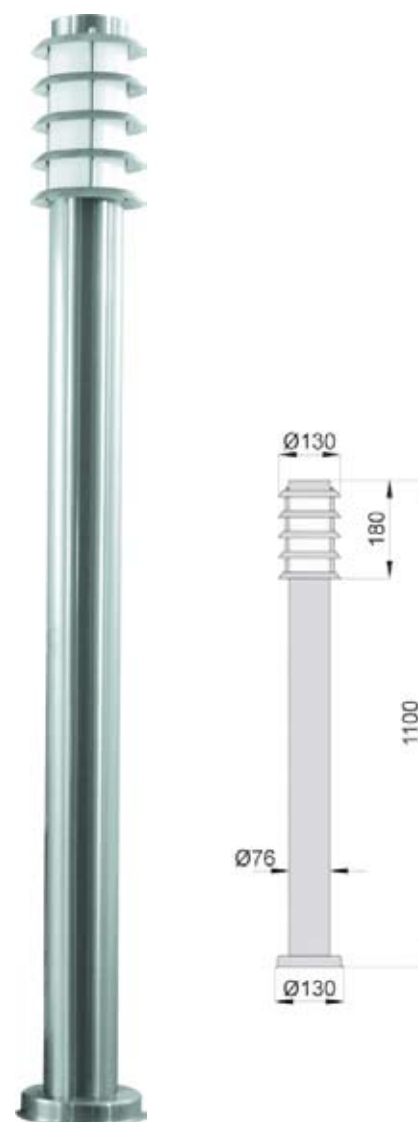
STELO 110B E 27, boja saten/hrom bela, materijal metal/plastika IP44
