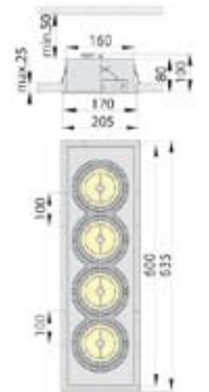
Unutrašnja svetiljka Pireo 410, 12V, aluminium
