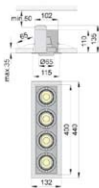
Unutrašnja svetiljka Tongo 400, 220V, aluminium
