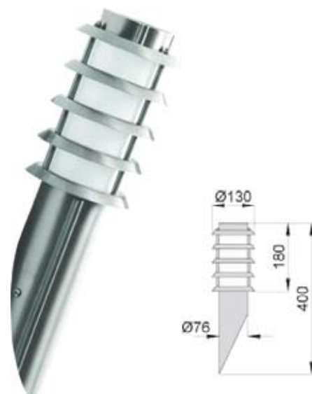
STELO 40B E 27, boja saten/hrom bela, materijal metal/plastika IP44
