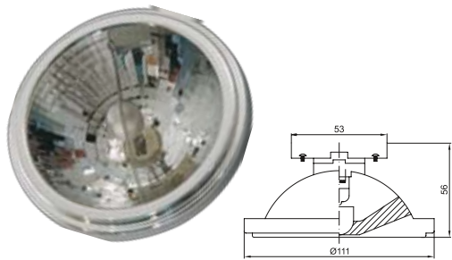
Halogena sijalica AR-111
