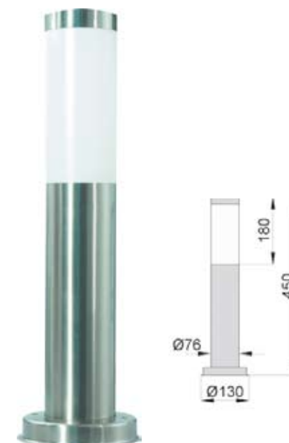
STELO 45A E 27, boja saten/hrom bela, materijal metal/plastika IP44
