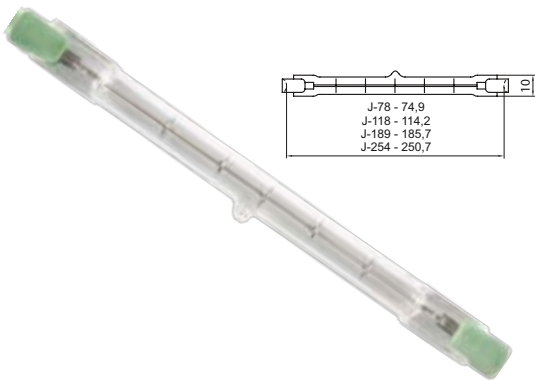
Halogena sijalica J-78/J-118
