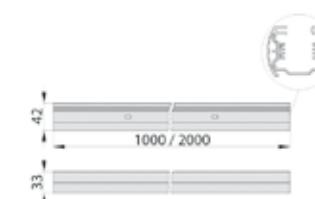
Scena TS | Aluminijum 1. TS-1m 2. TS-2m
