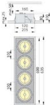
Unutrašnja svetiljka Paseo 410, 12V, aluminium
