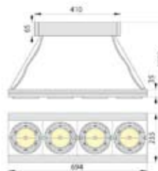
Unutrašnja svetiljka Lavado 410H, 220V, aluminium
